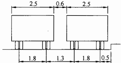
(6) 汽车荷载的横向布置
